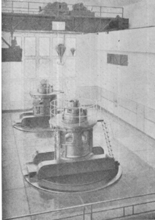
Salle des machines de l'usine d'El Kansera entièrement équipée par la Sté Als-Thom
