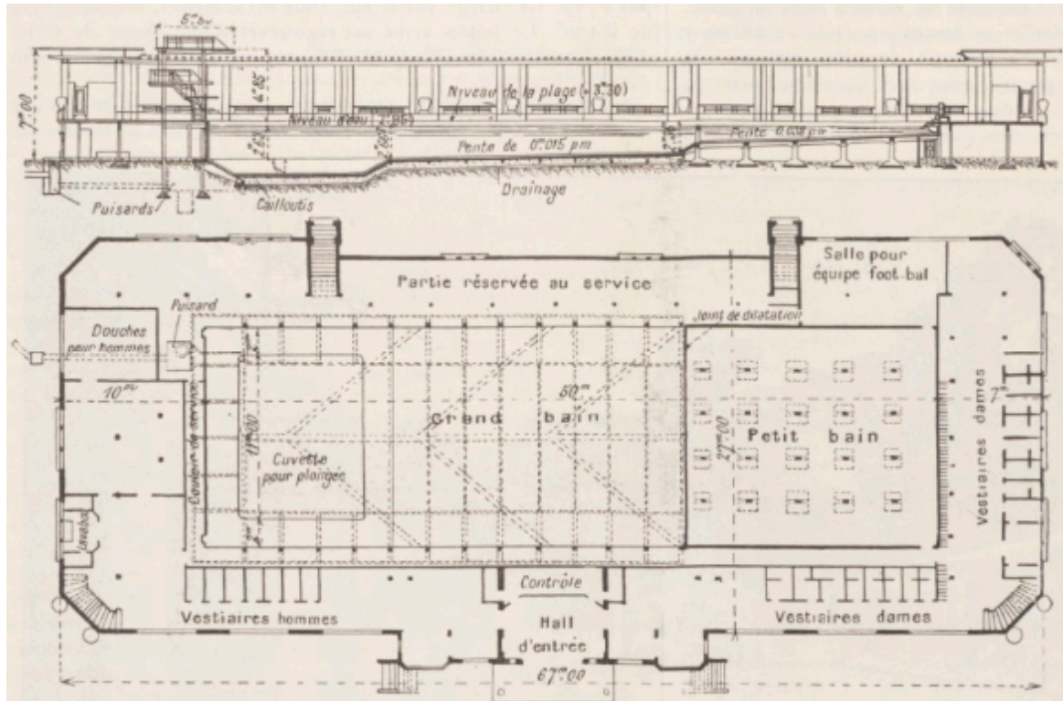
FIG. 2 et 3. — Coupe longitudinale et plan de la piscine de Saïgon.
