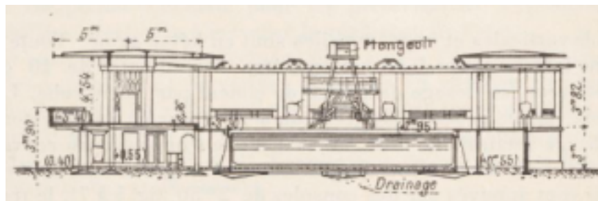
FIG. 4. — Coupe transversale de la piscine.
