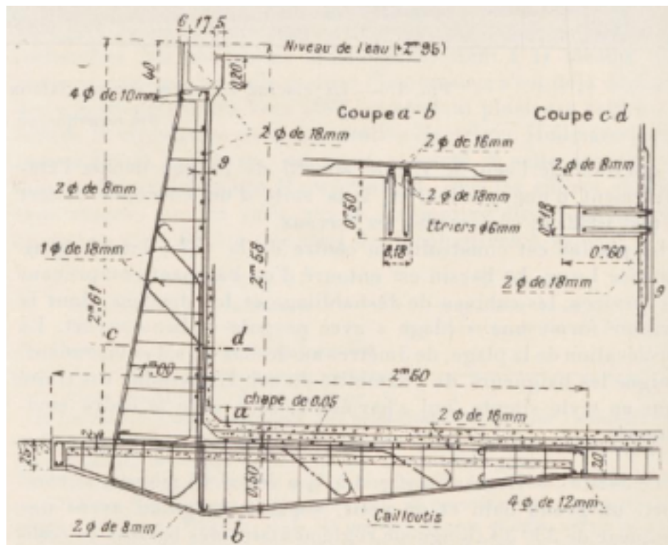
FIG. 5 à 7. — Coupe verticale et détails d'une console formant soutènement de la paroi verticale du grand bassin
