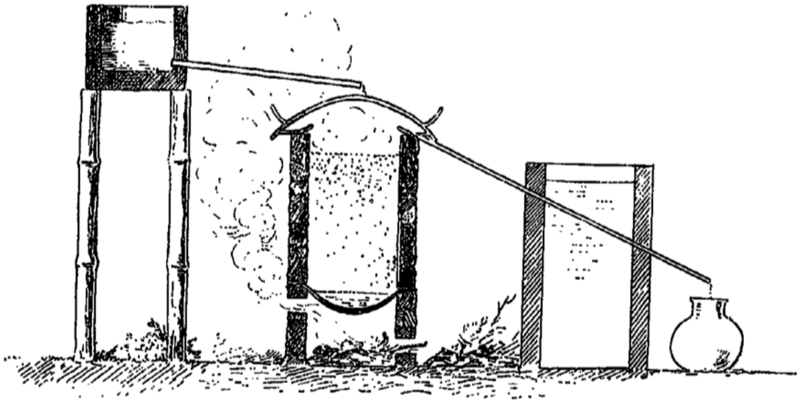
Appareil à distiller l'huile de badiane. — Dessin d'Eug. Burnand, d'après un croquis de l'auteur.
