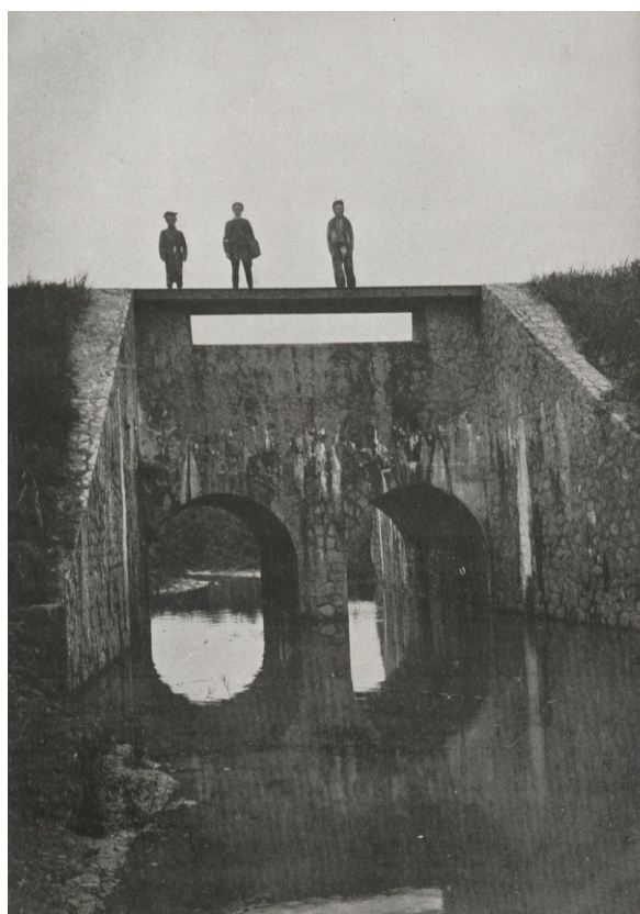
Irrigation de Kep. — Pont-canal et déversoir.
