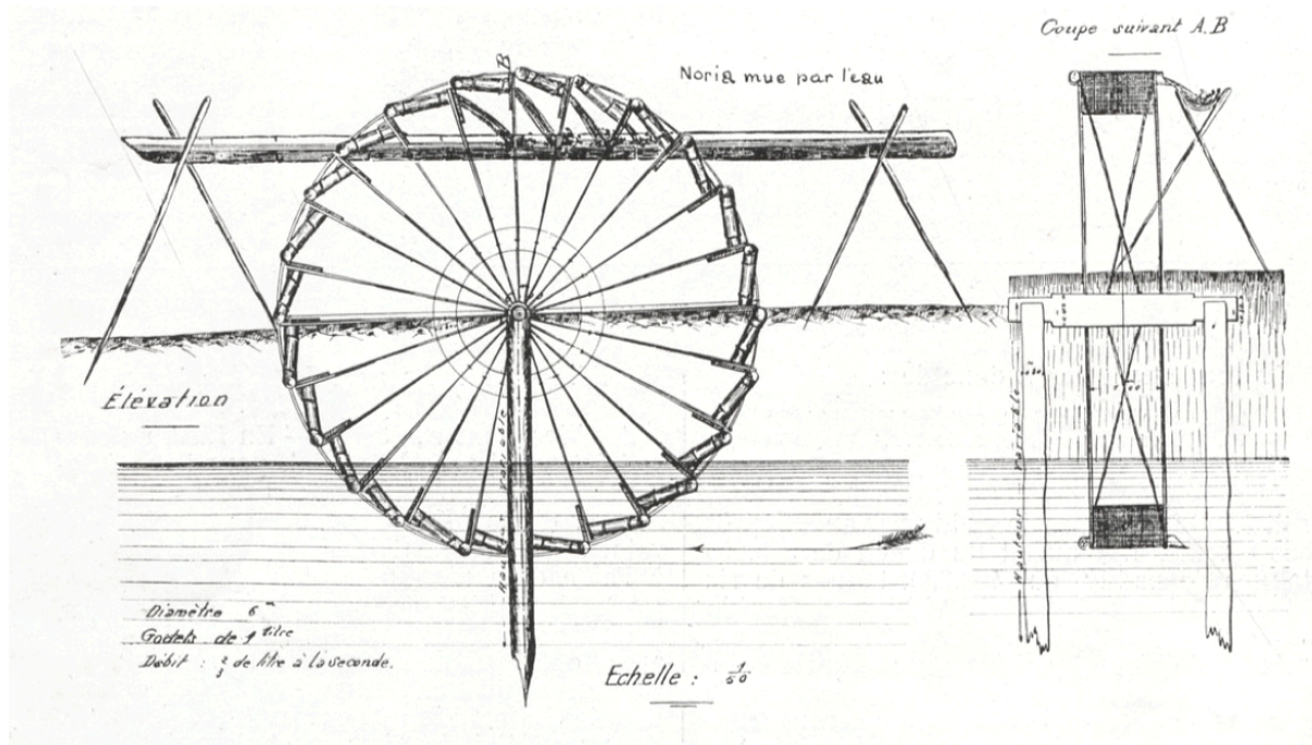
Noria mue par l'eau
